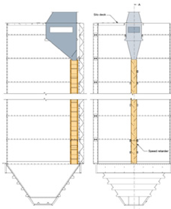
Каскад с дозирующим бункером
