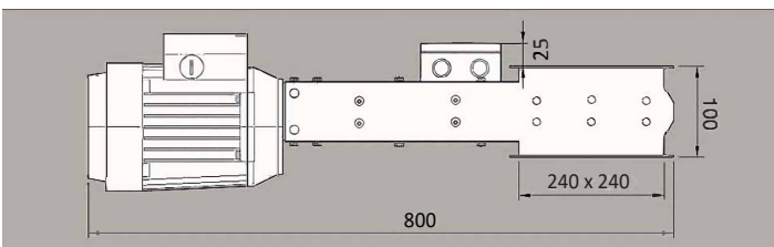
SKT79 Motorised
